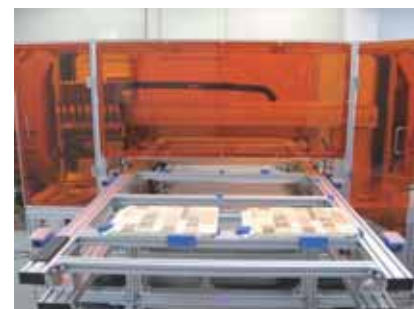
装置正面：搬送部イメージ ソリ防止の為に治具がついています。
